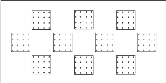
Posicionamiento de los puntos LED detrás de la tela ETTLIN LUX® Distancia de más o menos 5 a 20 cm
